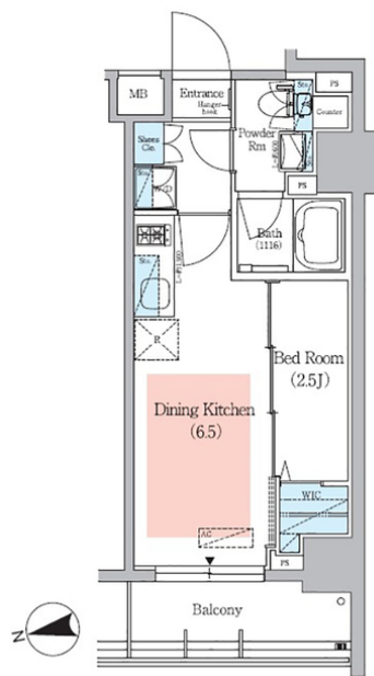
間取り図
